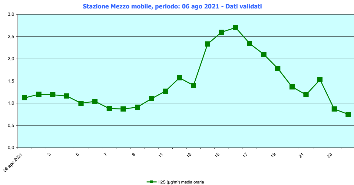
Figura 8: concentrazione (µg/m 3 ) media oraria di H 2 S
