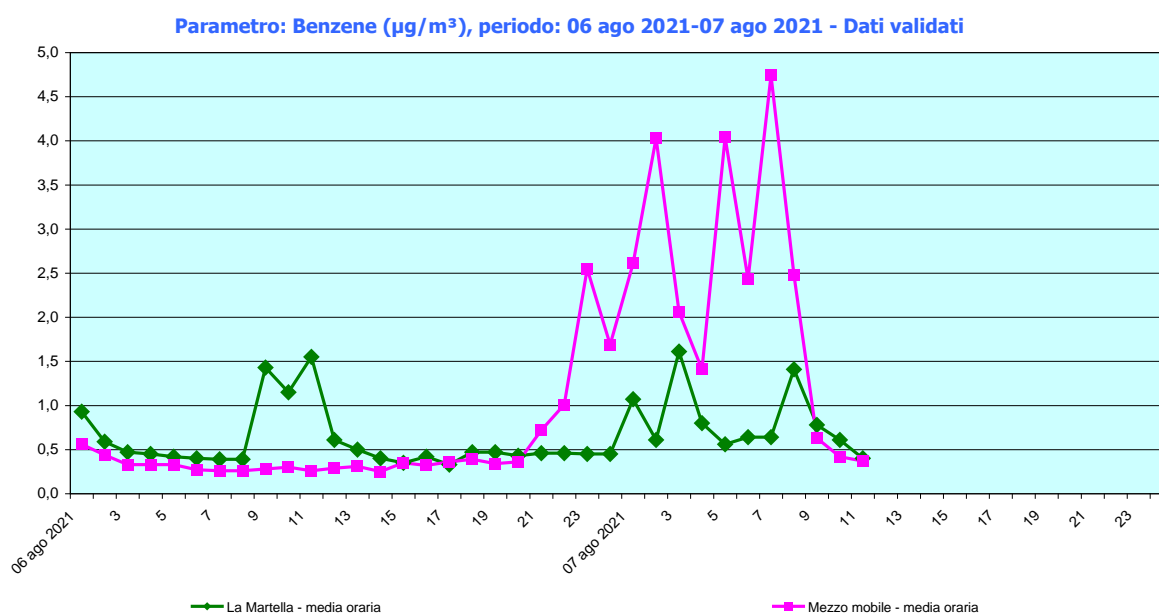
Figura 6 concentrazione (µg/m 3 ) media oraria di Benzene
